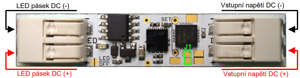
Obr.1 - Zapojení vývodů modulu
