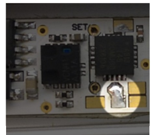
Obr.3 - Propojka J1
