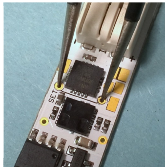
Obr.2 - Nastavení režimu
